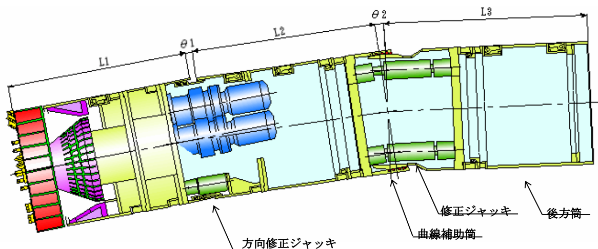
曲線補助筒仕様
